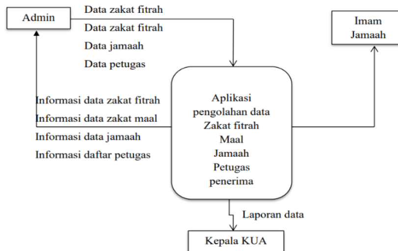
Gambar 3. DFD Sistem yang di usulkan
