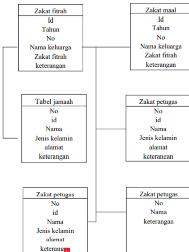
Gambar 4. Relasi Antar Tabel dalam database
