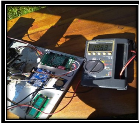
Gambar 4.15 Pengukuran Tegangan Panel Surya
