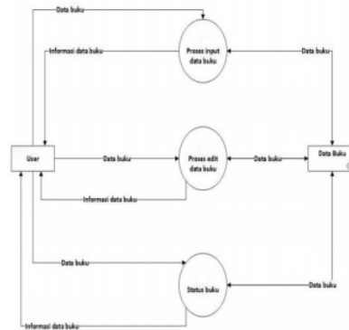
Gambar 5. Diagram level 2 proses mengolah data buku
