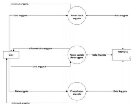
Gambar 4. Diagram level 2 mengolah data anggota
