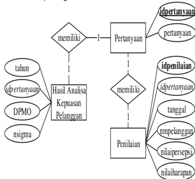
Gambar 3. ERD
