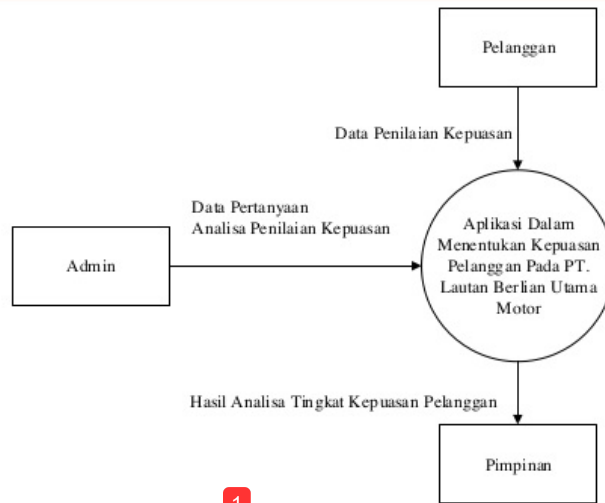
1 Gambar 1. Diagram Konteks
