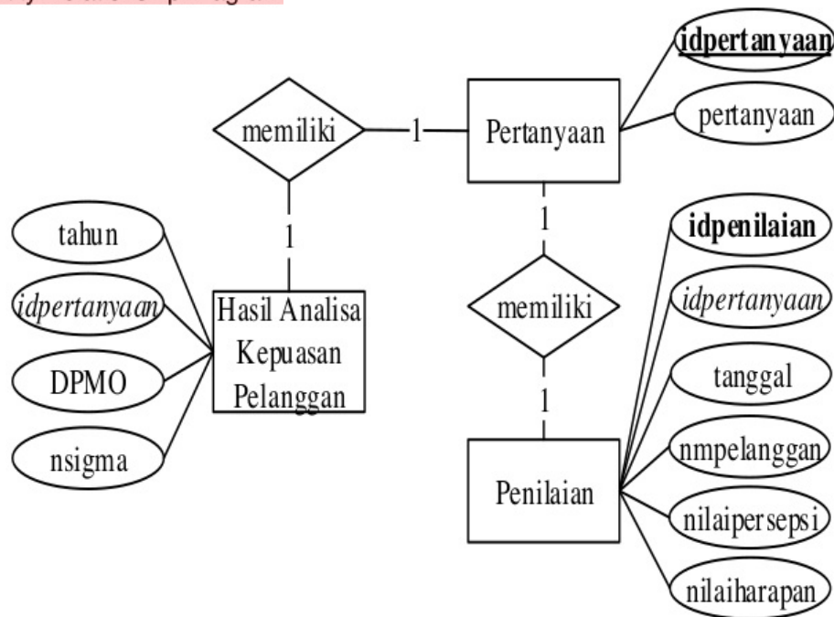
Gambar 3. ERD
