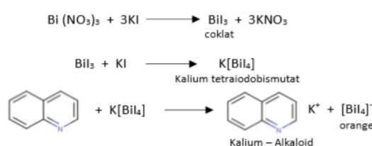
Gambar 1. Reaksi Uji Dragendroff
