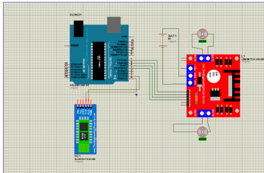
Gambar3RangkaianAlat
