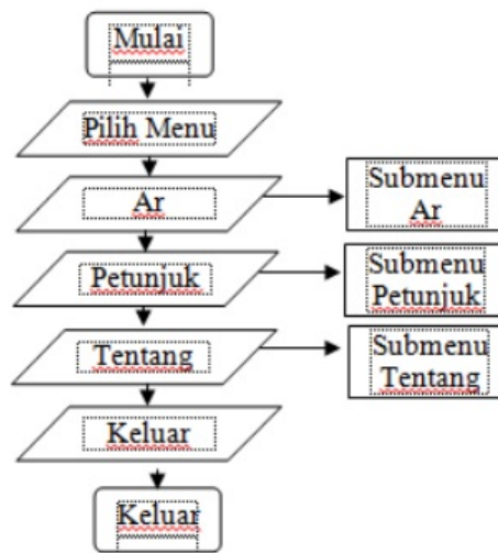
Gambar 10 Flowchart Aplikasi
