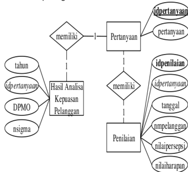
Gambar 3. ERD
