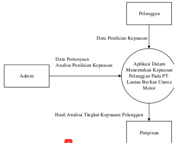
Gambar 1. Diagram Konteks
