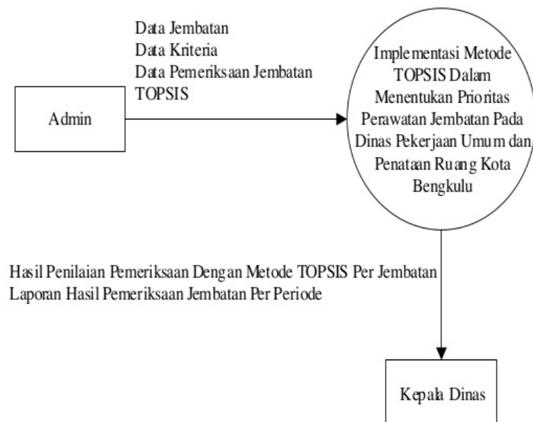
Gambar 2 .Diagram Konteks
